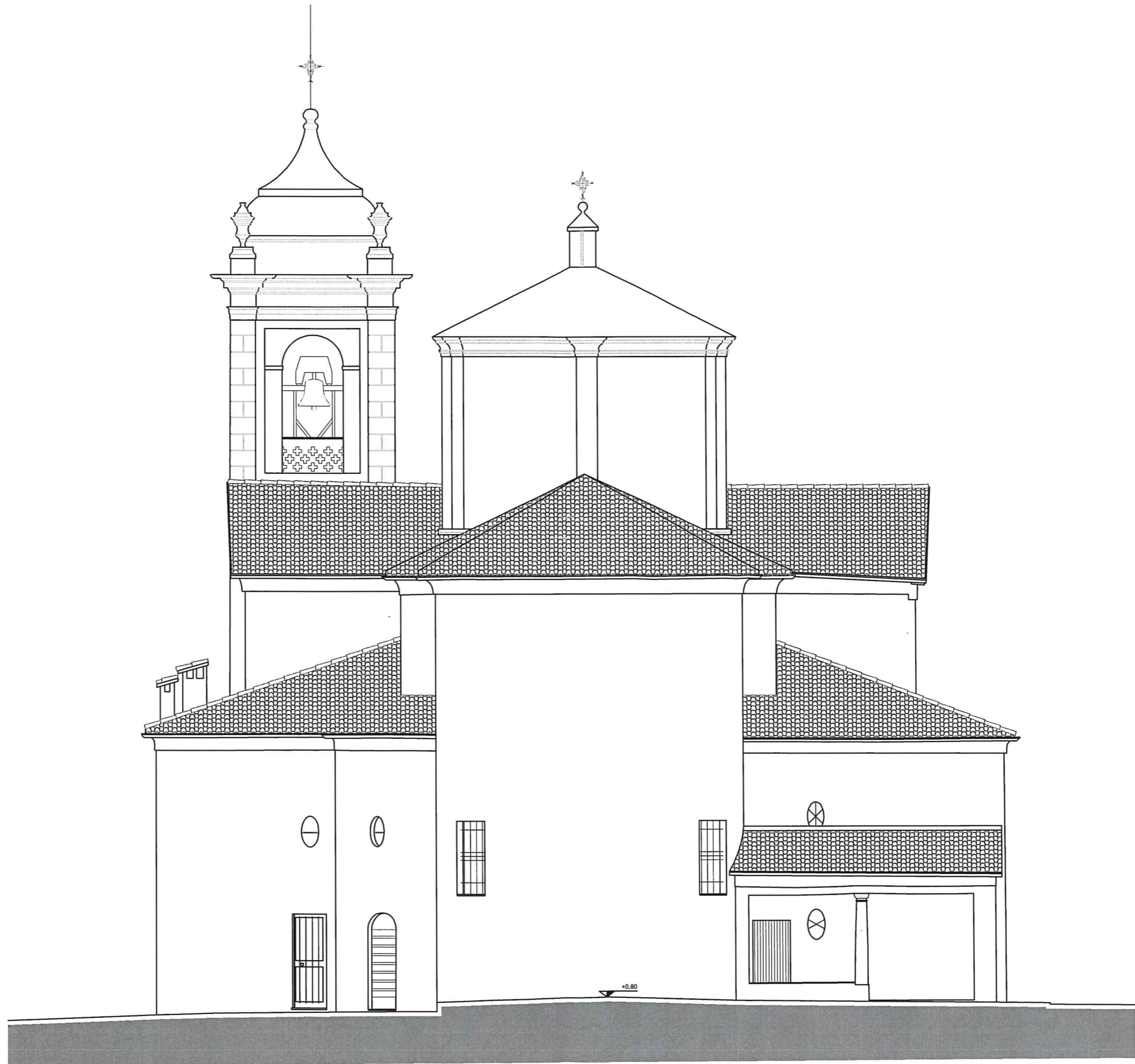
Prospetto Ovest
