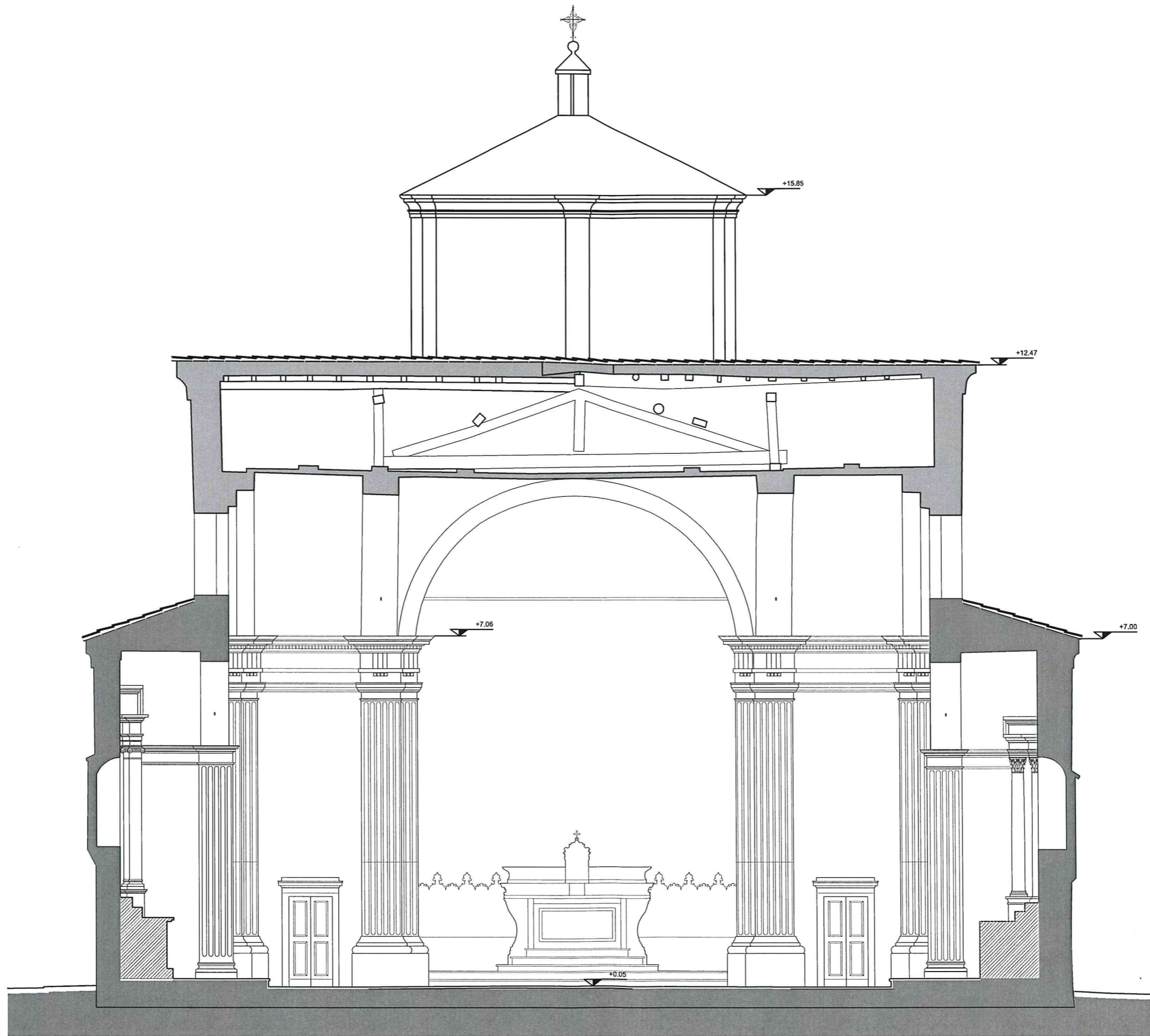
Sezione C
